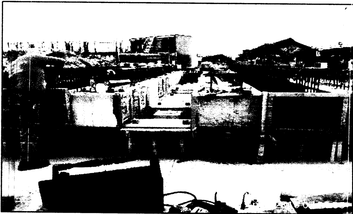
Imagen N°3: La excavadora tipo oruga está limpiando el área para colocar las estructuras de lozas para la construcción de las vigas longitudinales para el muelle.
