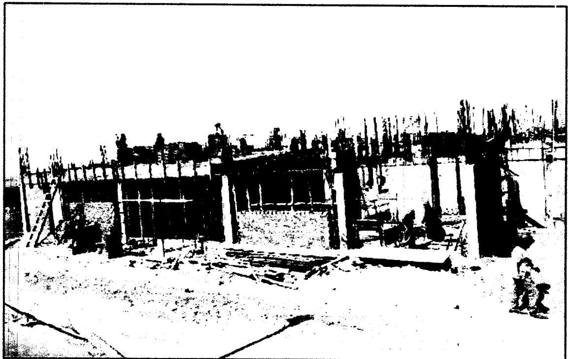
imagen N°7: A la vista de la imagen se aprecia a los trabajadores que se está haciendo trabajos con sus EPP's completos, colocando los ladrillos en el techo en la zona de Osmosis
